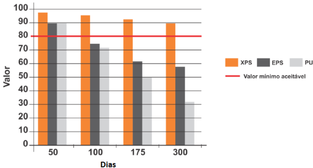
Valor de Condutividade Térmica durante 300 dias de imersão em água
