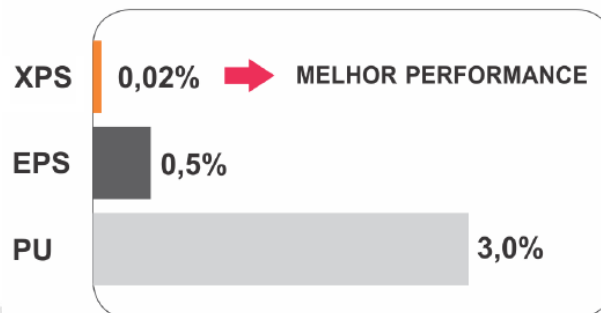
Porcentagem de absorção de água por volume
